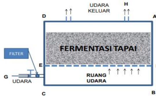
Gambar 1. Denah Alat Fermentasi
