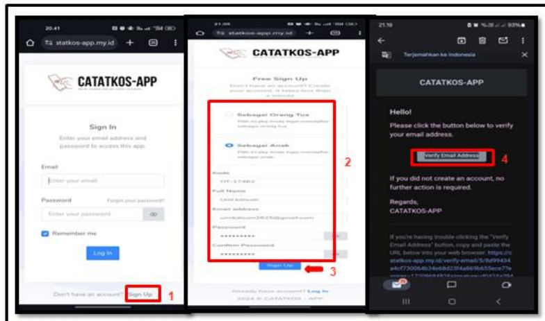
Gambar 3: daftar akun
