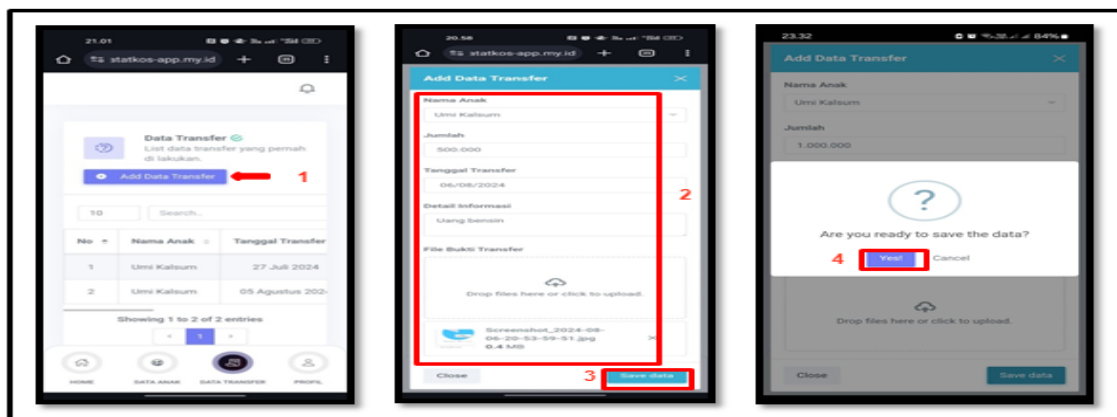
Gambar 4: pencatatan pemasukan
