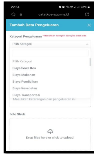
Gambar 6: pilihan pengeluaran
