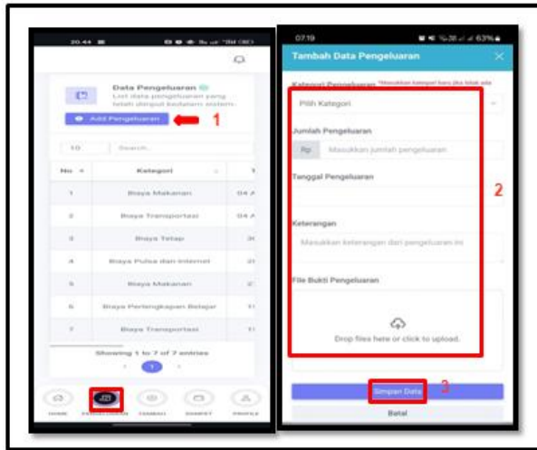
Gambar 5: pencatatan pengeluaran
