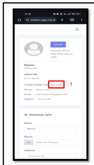
Gambar 2: kode anak
